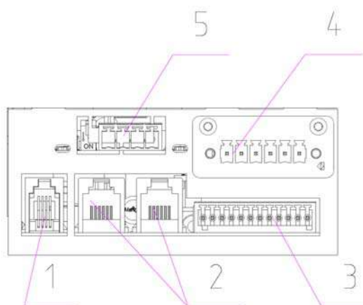
Рисунок 1.1 – Установка питания постоянного тока Штиль PS48-0160-3U, ver.2 3 . Вид с фронтальной стороны
