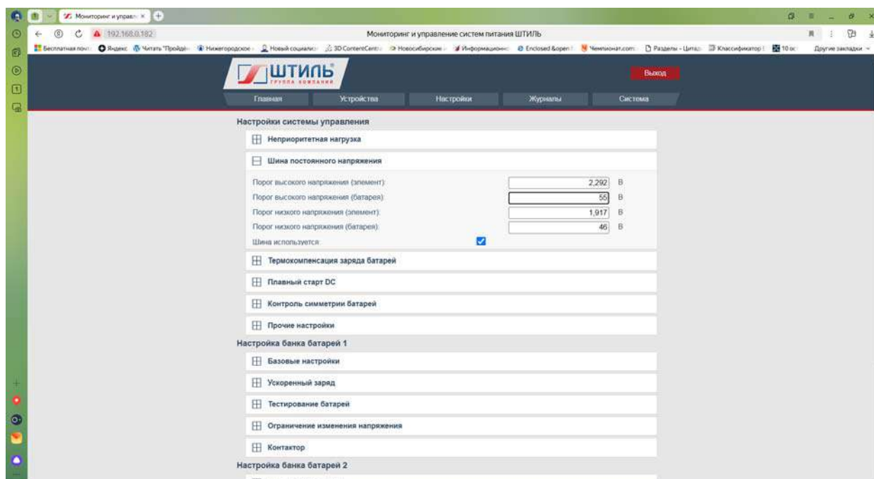
Рисунок Б1 - Пороги высокого и низкого напряжения
