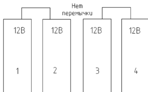
Рисунок 2.1 – Рекомендуемая конфигурация сборки АБ перед подключением
