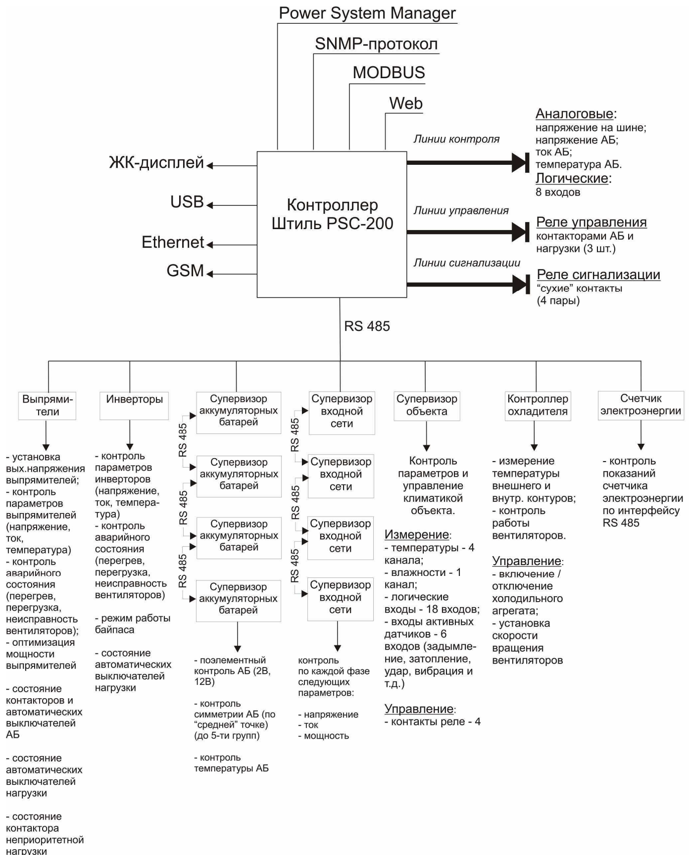
Рисунок 1.3 - Структура контроллера Штиль PSC-200 (максимальная конфигурация)
