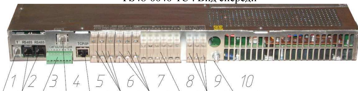
Рисунок 1.1 - Установка питания постоянного тока Штиль PS48-0040-1U . Вид спереди
