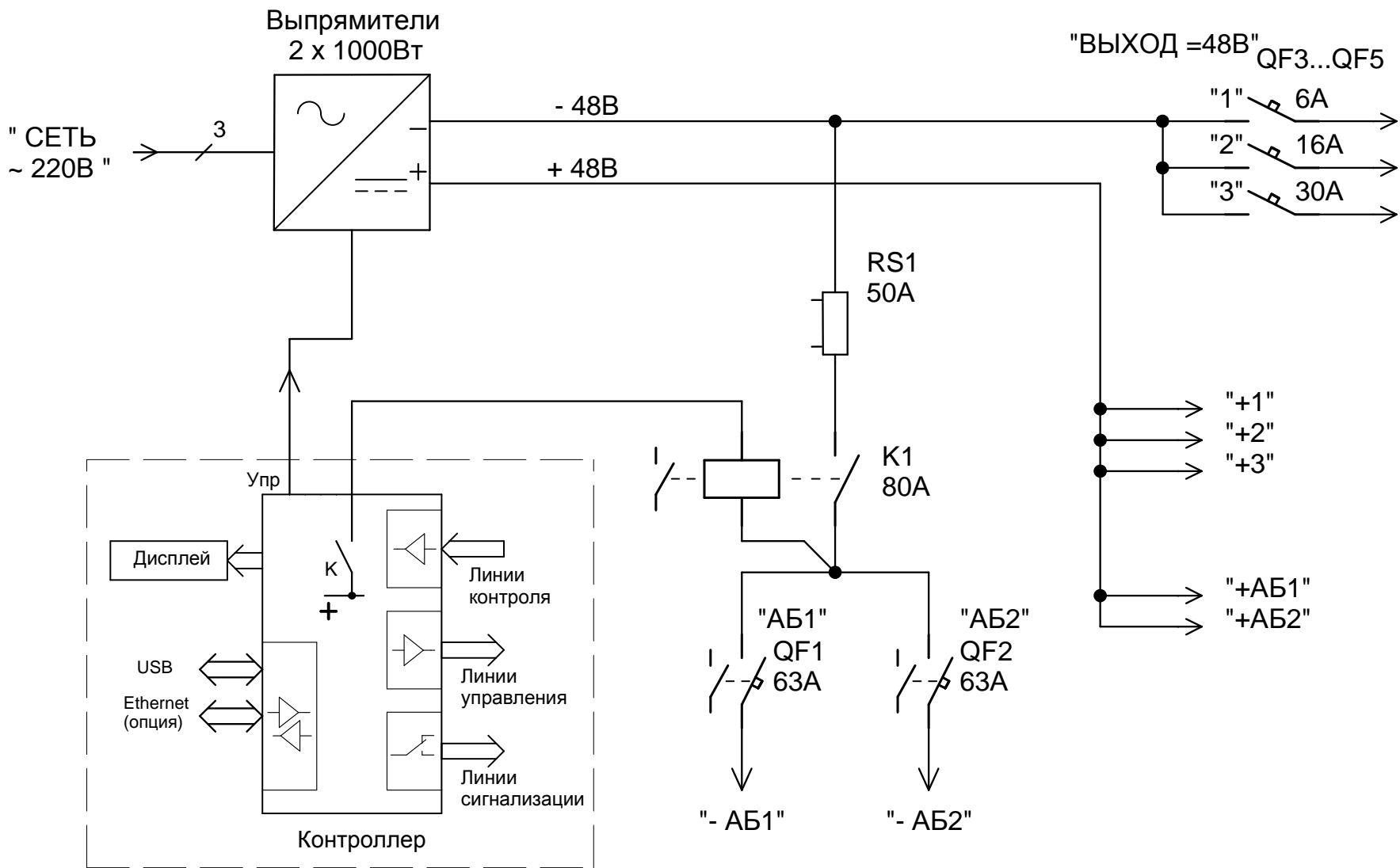
ПРИЛОЖЕНИЕ Б ФУНКЦИОНАЛЬНАЯ СХЕМА ИЗДЕЛИЯ
