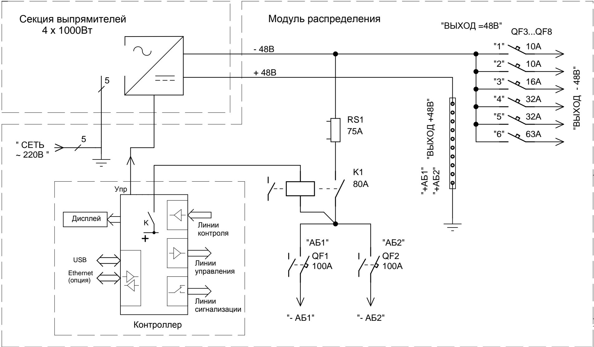
ПРИЛОЖЕНИЕ Б ПРИНЦИПИАЛЬНАЯ СХЕМА ИЗДЕЛИЯ
