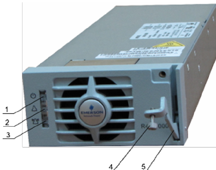
1 – индикатор «Работа», 2 – индикатор «Авария», 3 – индикатор «Аварийное отключение», 4 – рукоятка, 5 – винт Рисунок 1.4 - Выпрямитель Emerson BML 440021/1
