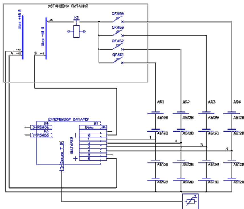
Рисунок 2.2 – Подключение модуля САБ. Контроль симметрии.
