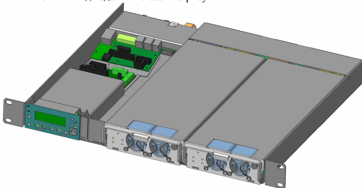
Рисунок 1.1 - Модульный каркас PS1000KM с инверторами PS48-60/1000К и контроллером Штиль PSC-200
